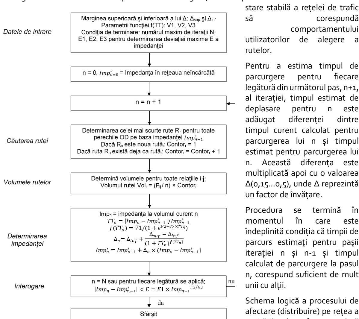
Figură 82 - Schema logică a metodei "Echilibru-Lohse" de afectare pe itinerarii
