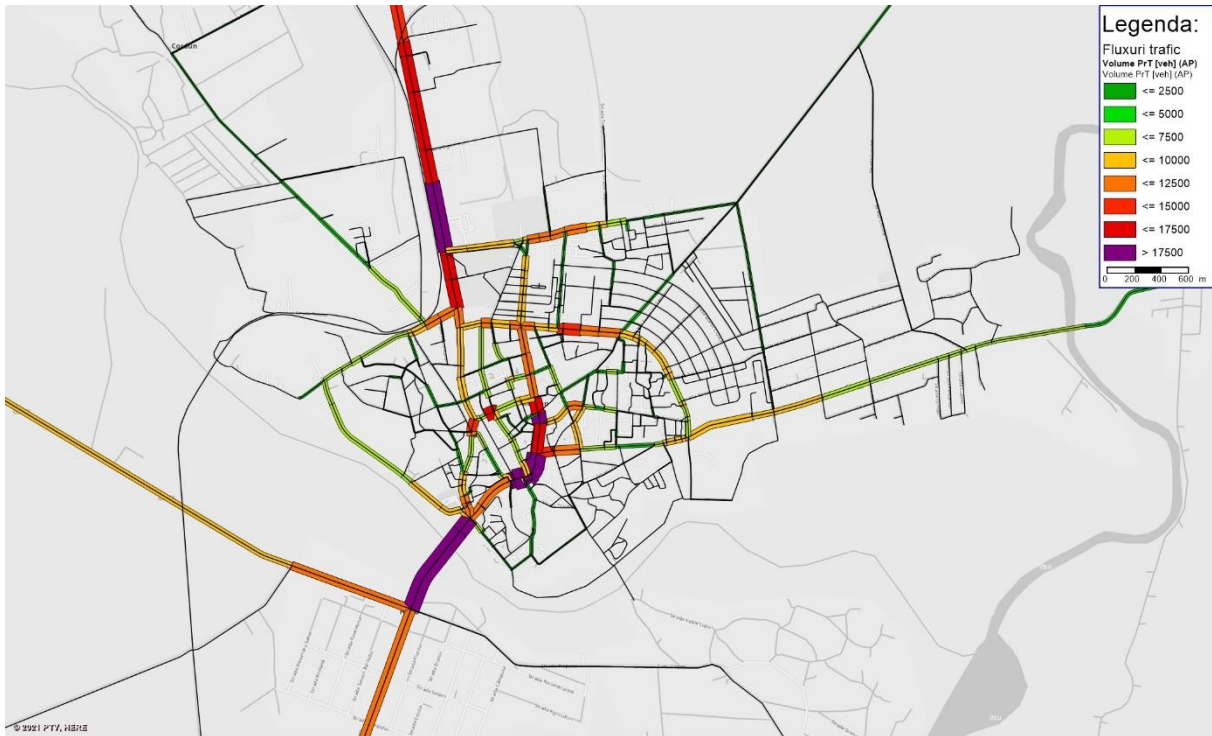
Figură 92 - Afectarea traficului, anul de bază 2021 Sursa: Analiza Consultantului asupra Modelului de Transport
