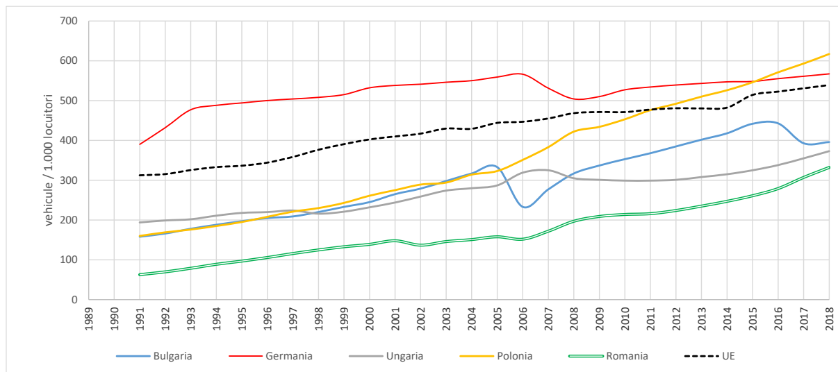
Figură 90 - Evoluția gradului de motorizare în România fata de media europeană (EU27) - turisme / 1.000 locuitori
