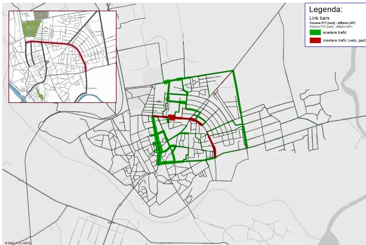
Figură 91 – Planșa „diferențe” a proiectului testat Co1 (anul 2030)
