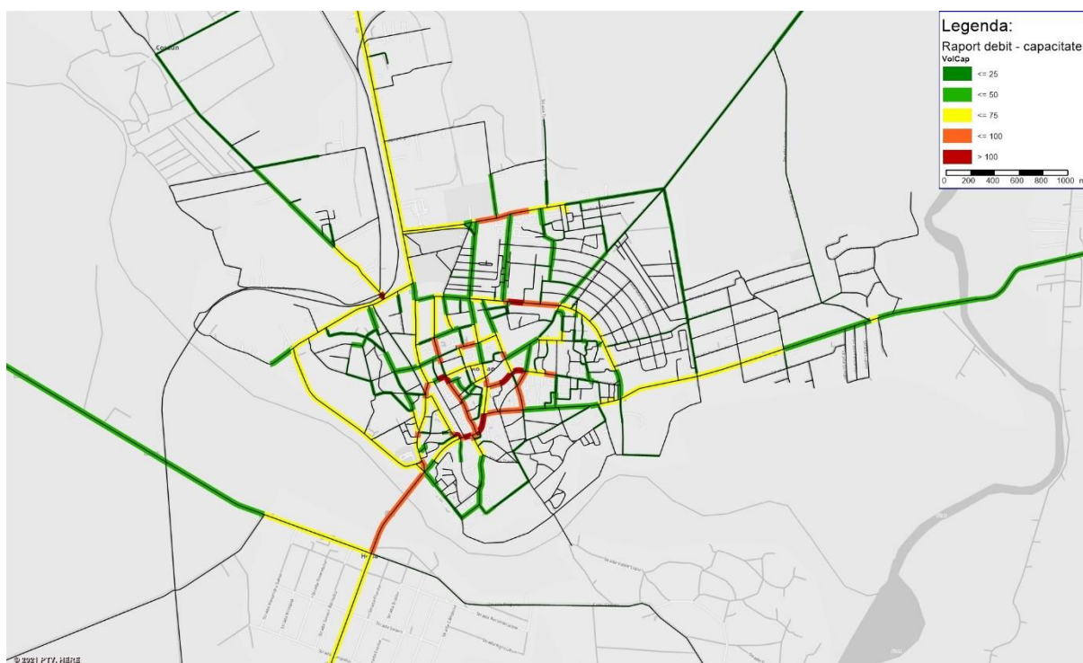
Figură 94 - Raportul debit-capacitate, anul de bază 2021, ora de vârf PM Sursa: Analiza Consultantului asupra Modelului de Transport
