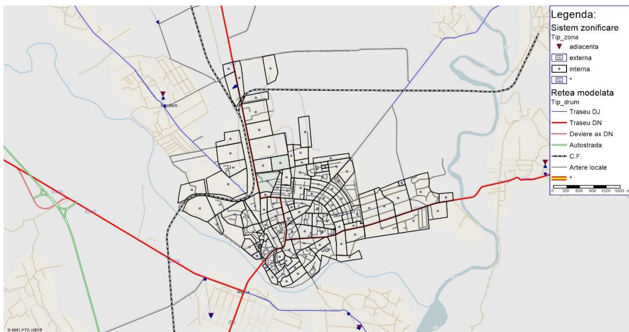
Figură 80 - Sistemul de zonificare intern folosit în cadrul modelului de trafic elaborat pentru municipiul Roman Sursa: Hartă realizată de consultant
