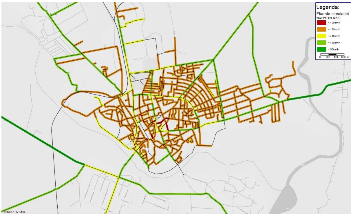
Figură 93 - Fluența circulației, anul de bază 2021 Sursa: Analiza Consultantului asupra Modelului de Transport
