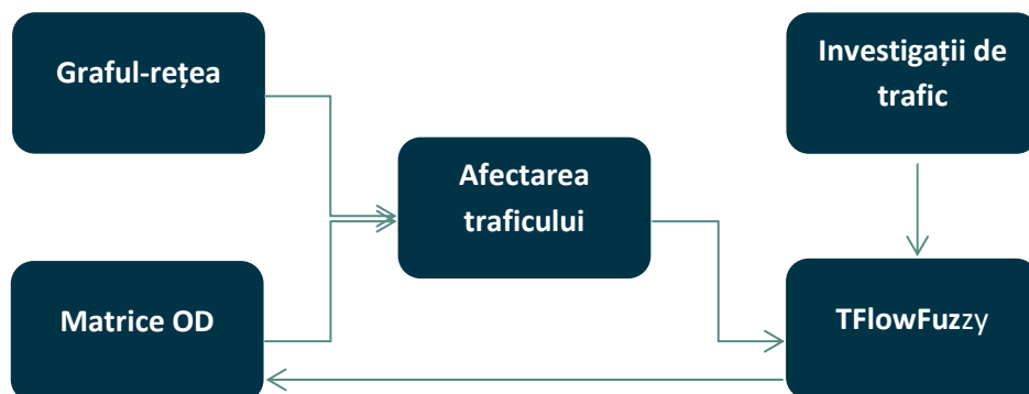
Figură 84 - Schemă a logică a procesului de calibrare utilizat
