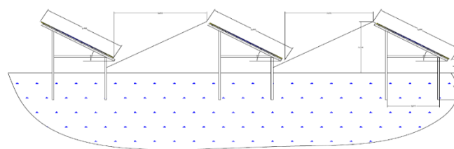
SECTIUNE AMPLASARE BATERII DE PANOURI FOTOVOLTAICE
