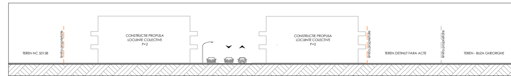
D2 Desfasurare stradala - Strada cocorului
