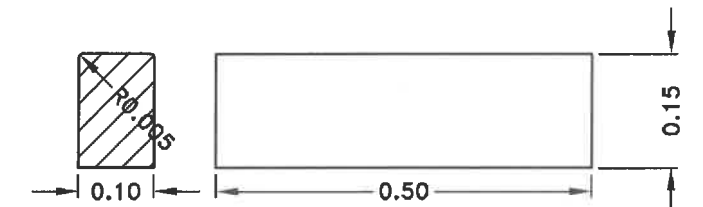
BORDURA B1x500/l/finisata SR EN 1340
